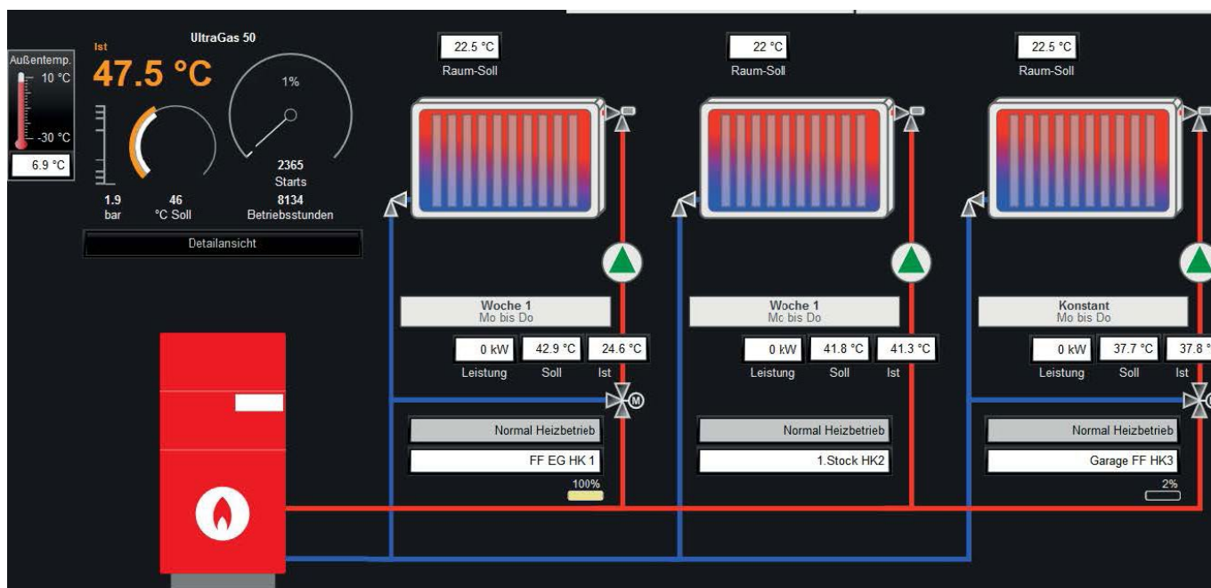
Visione d'impianto per edificio commerciale con la regolazione HovalSupervisor.
