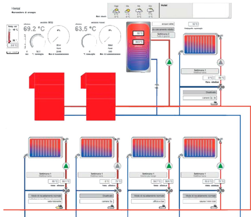
Visione d'esempio di revamping di una centrale termica tramite HovalSupervisor.
