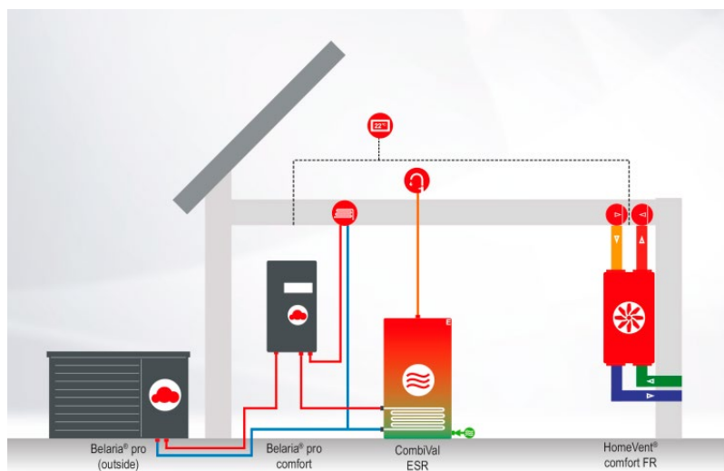
Schema stilizzato con pompa di calore Belaria® e sistema di VMC HomeVent® inerente al settore residenziale.
